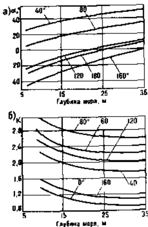
Рисунок 1 - Изменение угла \alpha_1 отклонения направления поверхностных течений (а) и ветрового коэффициента K (б) в зависимости от направления ветра относительно берега и глубины моря (мелководная зона)
